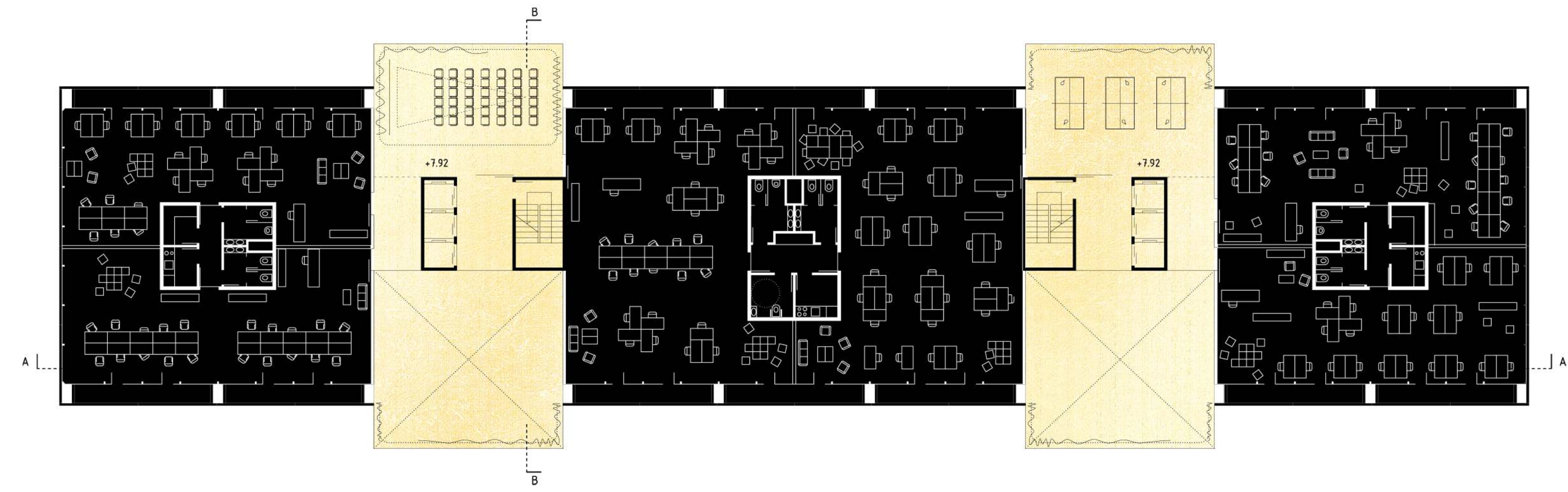
TLOCRT KARAKTERISTIČNOG KATA 2
