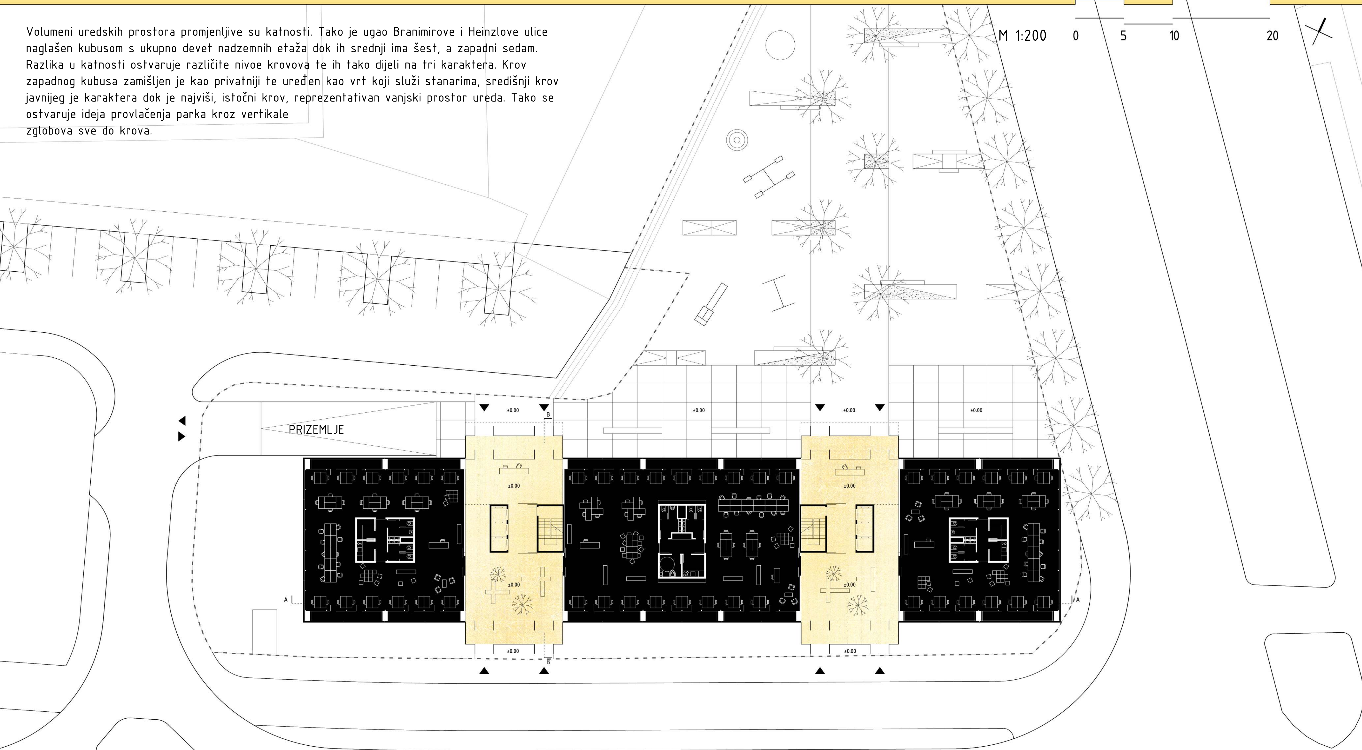
TLOCRT PRIZEMLJA
