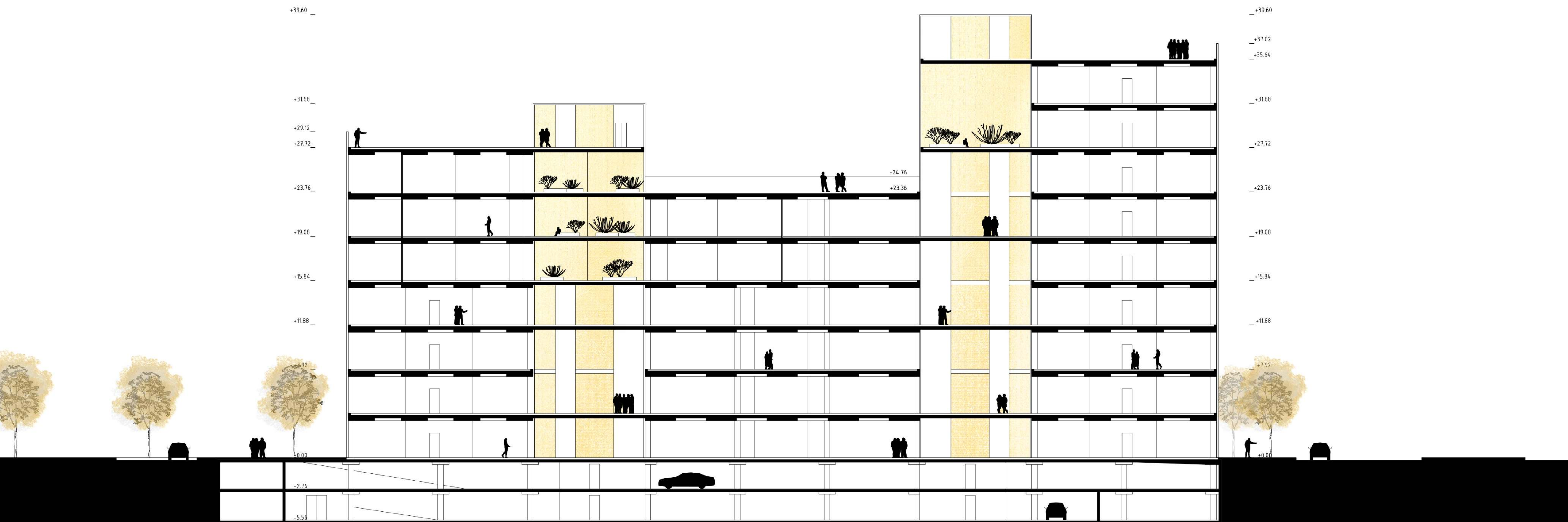
PRESJEK A-A
