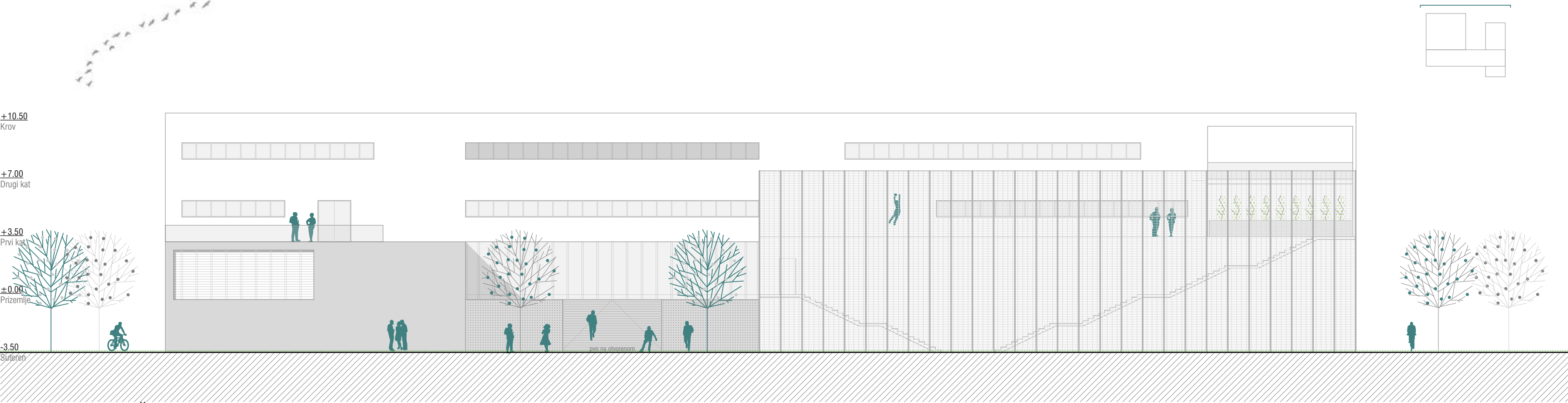
SJEVERNO PROČELJE_M 1:200
