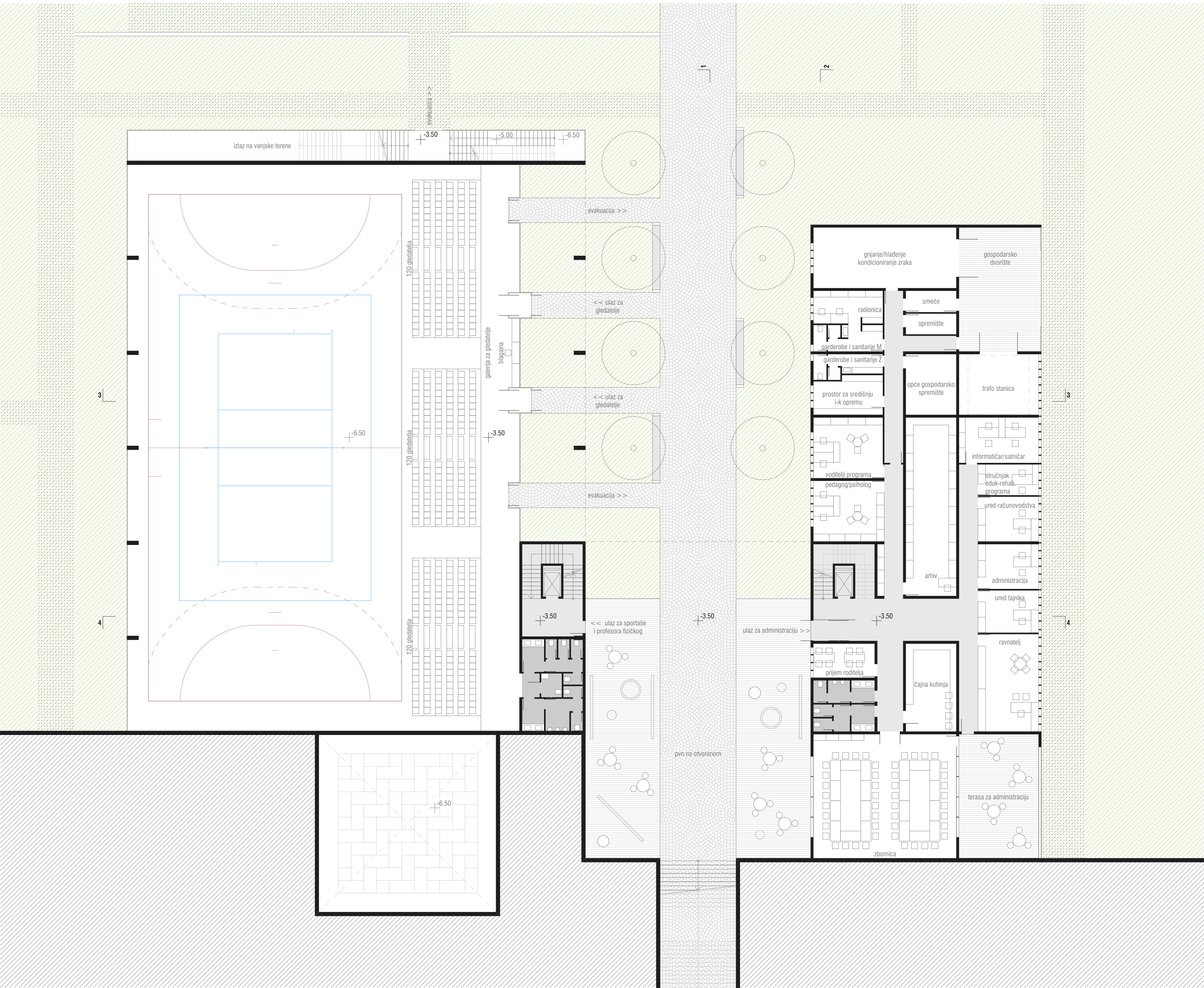
TLOCRT SUTERENA_M 1:200
